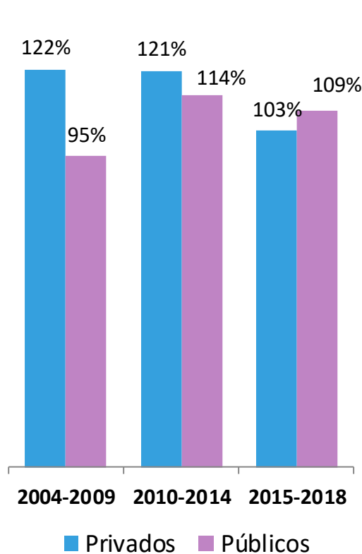
Tasa reclutamiento (%)
