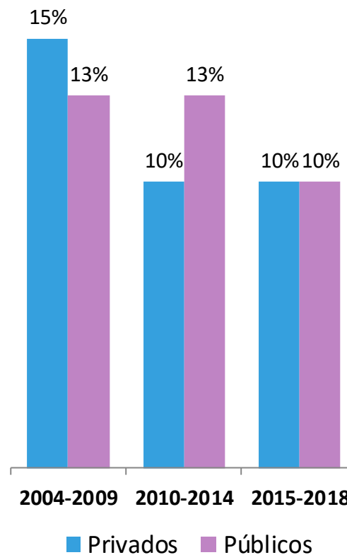
Sin reclutamiento (%)
