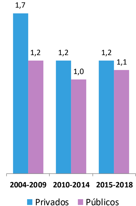
Velocidad (pac/mes)
